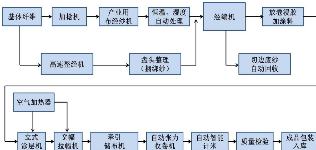
图2 纤维复合土工格栅工艺流程
