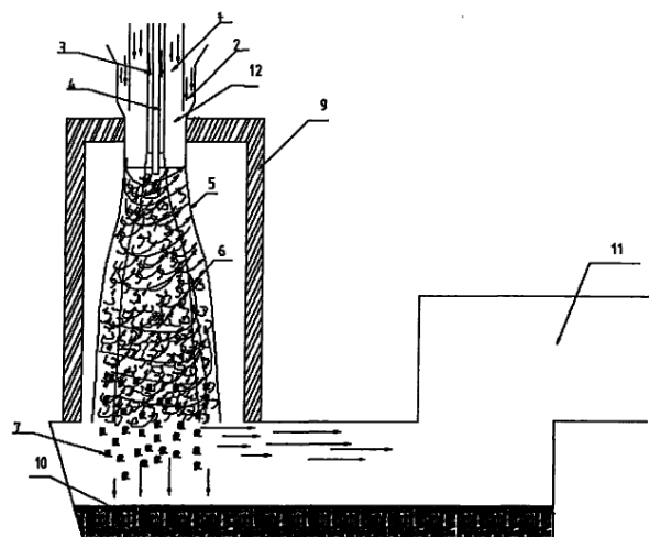
1-富氧空气，2-粉状物料，3-脉动氧气，4-脉动燃料枪，5-高旋流体，6-脉动紊流， 7-分离出的液滴，8-高温烟气，9-反应器，10-熔池，11-排烟道，12-脉动旋流喷嘴
