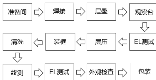
图 2 光伏组件工艺流程图
