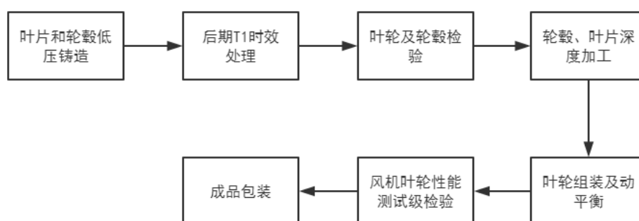
图 2 风机及叶轮的制造工艺流程图
