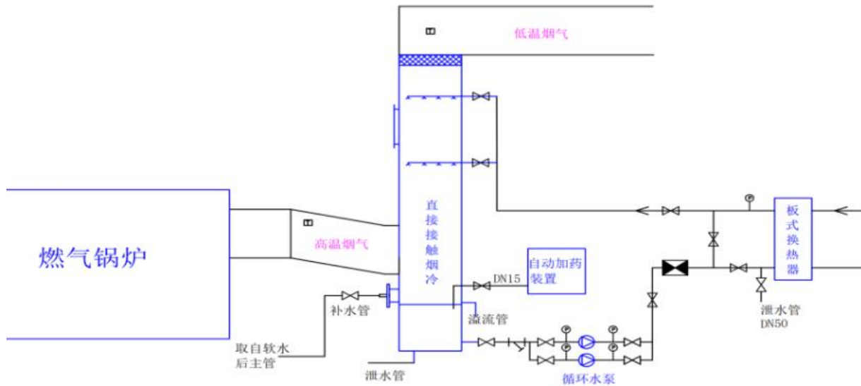
直接接触式烟气余热回收系统系统图
