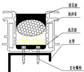
建筑光伏构件系统防水方案
